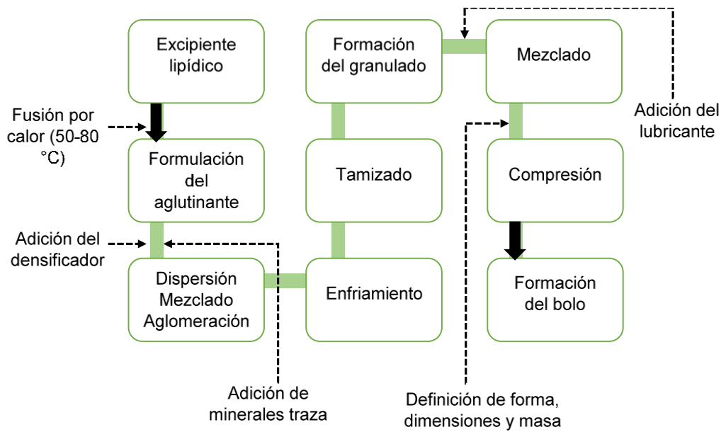
Figura 1: Diagrama del proceso de elaboración de bolos intrarruminales de selenio por el método de granulación por fusión
